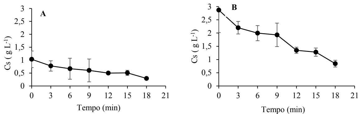
Figura 09. Relação da concentração de sedimentos e tempo de teste após o início do escoamento em Luvisso solo com cobertura vegetal sob chuva de 60 mm h -1 (A) e 100 mm h -1 (B). (Fonte: Elaborada pela autora a partir da coleta de dados experimentais)
