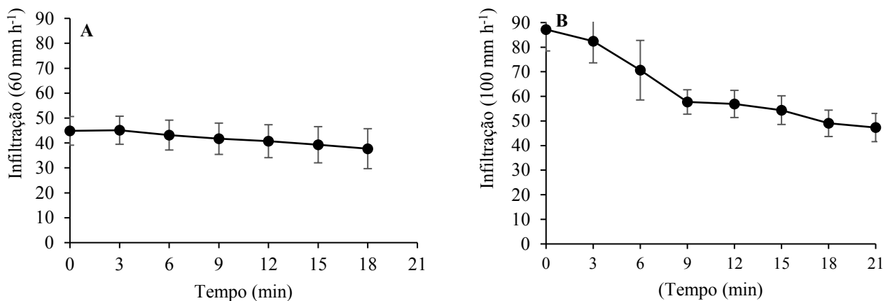
Figura 13. Relação da infiltração e tempo de teste após o início do escoamento em Luvisolo com cobertura vegetal sob chuva de 60 mm h -1 (A) e 100 mm h -1 (B). (Fonte: Elaborada pela autora a partir da coleta de dados experimentais)
