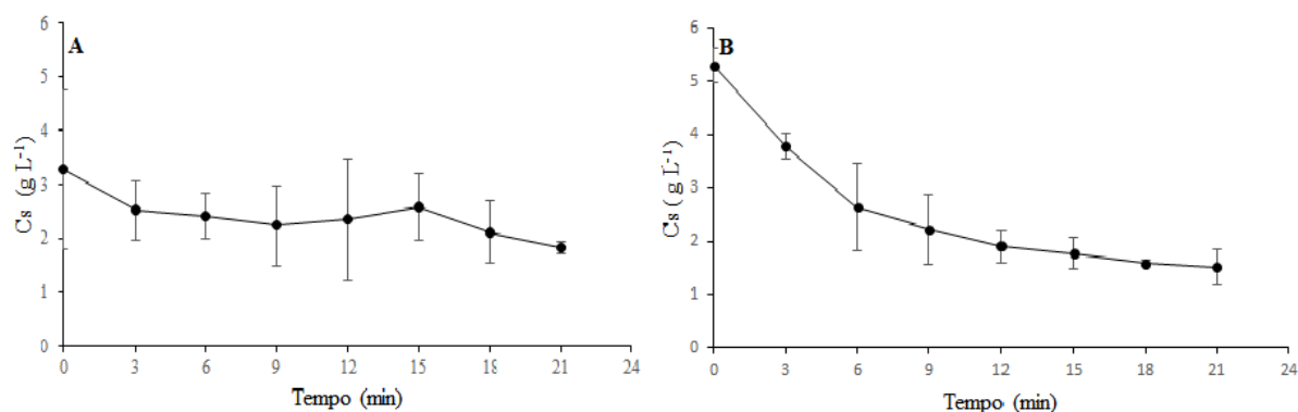
Figura 10. Relação da concentração de sedimentos e tempo de teste após o início do escoamento em Luvisso solo sem cobertura vegetal sob chuva de 60 mm h -1 (A) e 100 mm h -1 (B). (Fonte: Elaborada pela autora a partir da coleta de dados experimentais)
